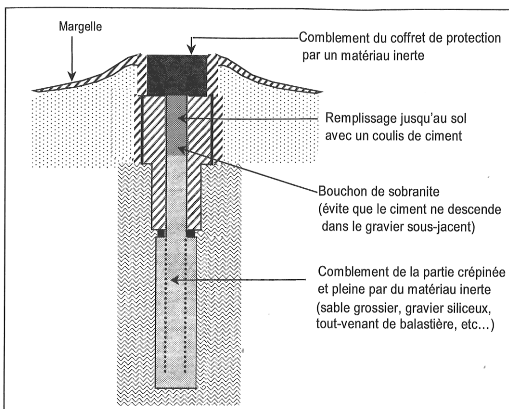
Illustration 24 Exemple d'un forage abandonné correctement comblé
