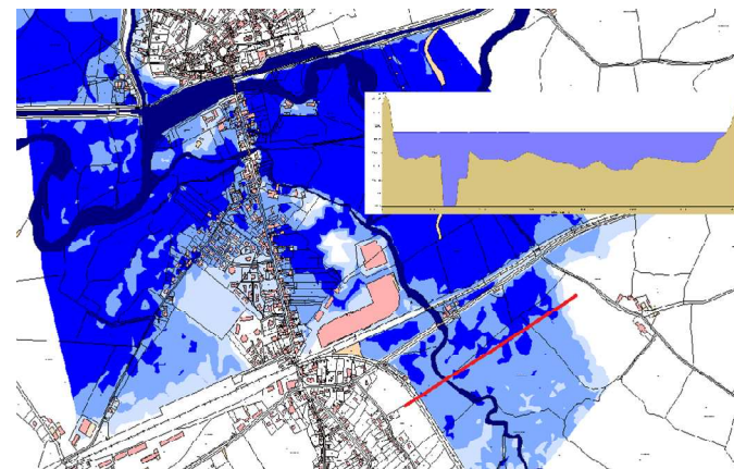
Figure 5: Vue en plan et profil en travers de la crue de 1866 à Cercy-la-Tour
