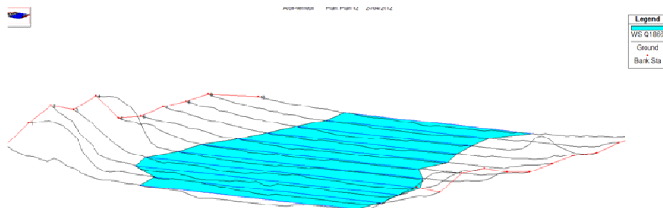
Figure 6: Modélisation filaire de l'Aron entre Cercy-la-Tour et Verneuil pour la crue de référence
