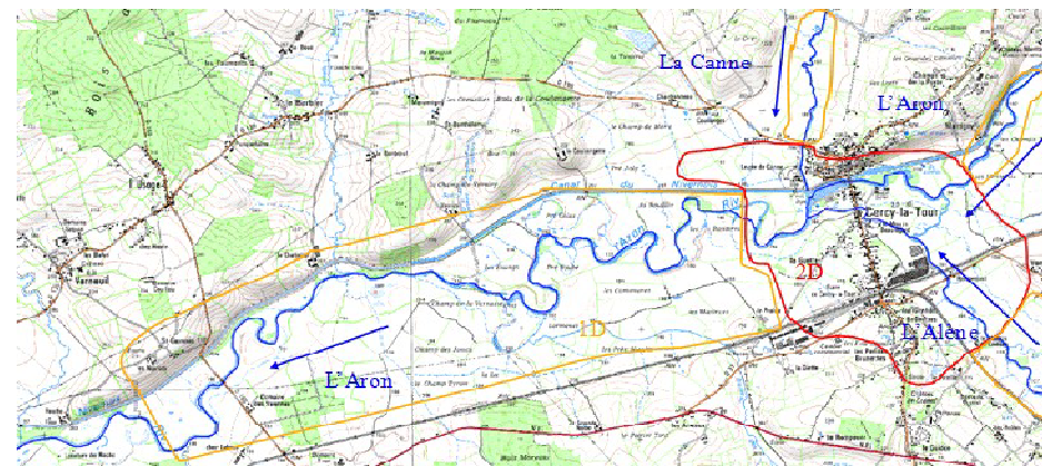
Figure 4: Zones modélisées sur les communes de Cergy-la-Tour et Verneuil (modélisation hydraulique bidimensionnelle en rouge et filaire en orange)
