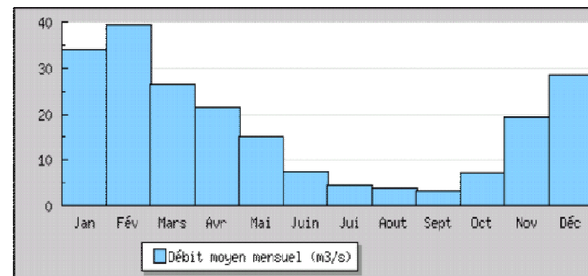
Figure 2: Débit moyen mensuel de l'Aron à Verneuil
