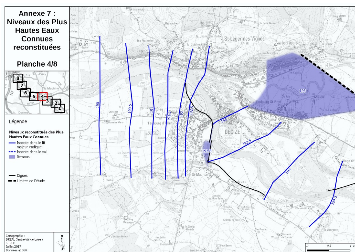
Reconstitution des isocotes finales
