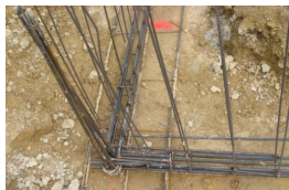
Noeud de chaînage - Continuité mécanique
