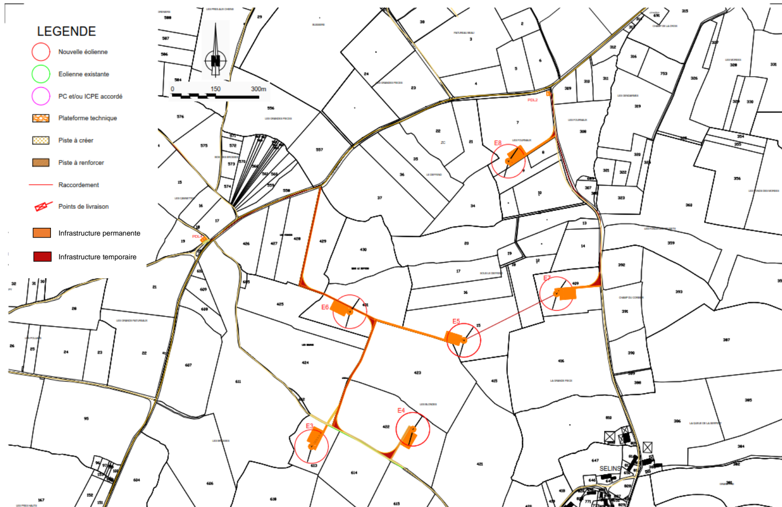
FIGURE 6 : PLAN D'IMPLANTATION DES EOLIENNES AVEC CHEMIN D'ACCES ET POSTES DE LIVRAISON
