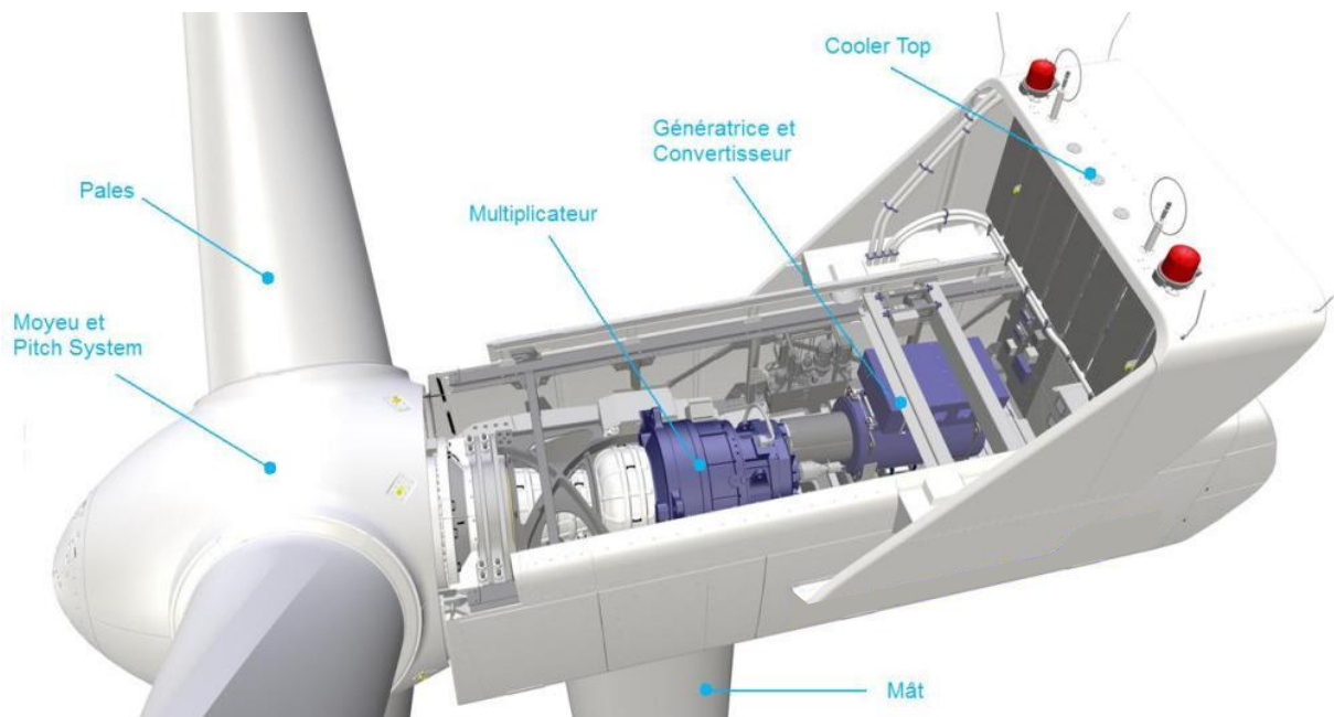
FIGURE 13 : SCHEMA DE LA NACELLE DE L'EOLIENNE
